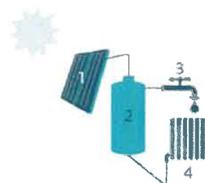
1 Zonnecollector | 2 Opslagvat zonneboiler | 3 Sanitair warm water | 4 Warmte-element voor ruimteverwarming (afhankelijk)
