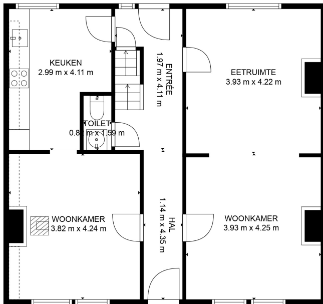
2. GELIJKVLOERS
