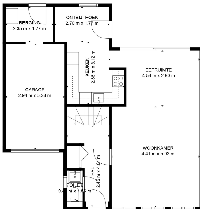
1. GELIJKVLOERS
