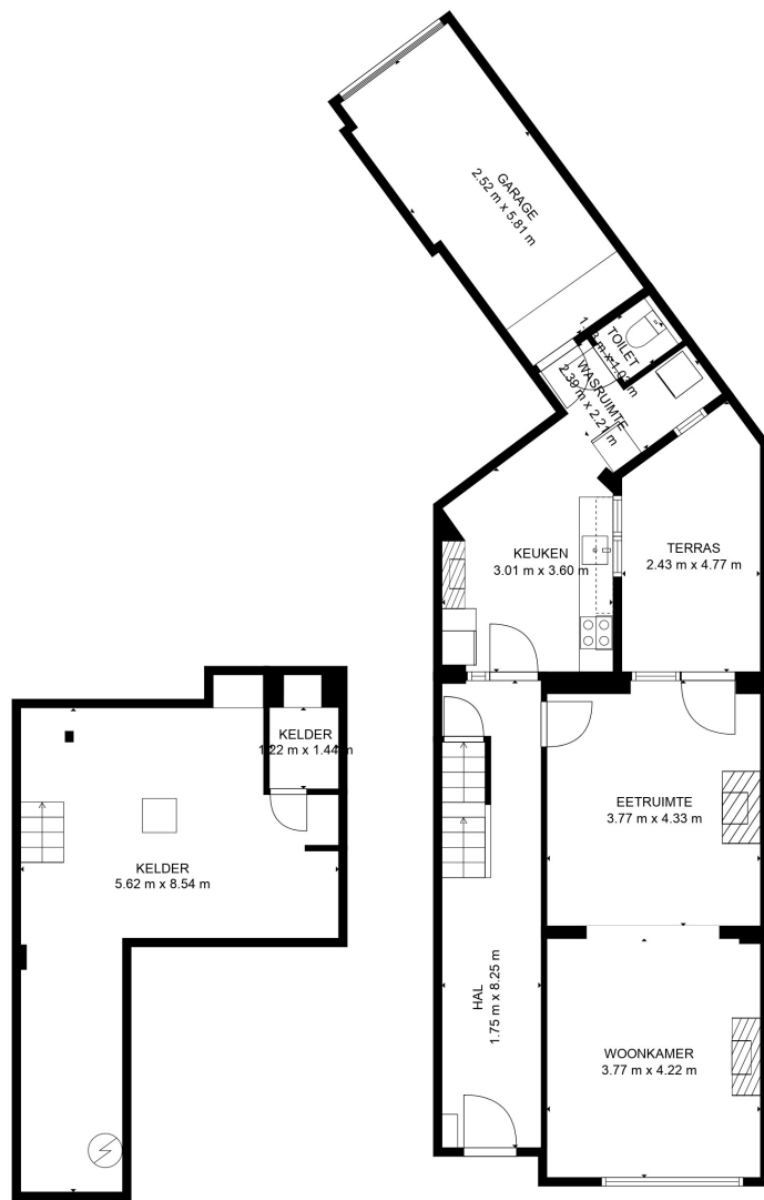
2. GELIJKVLOERS
