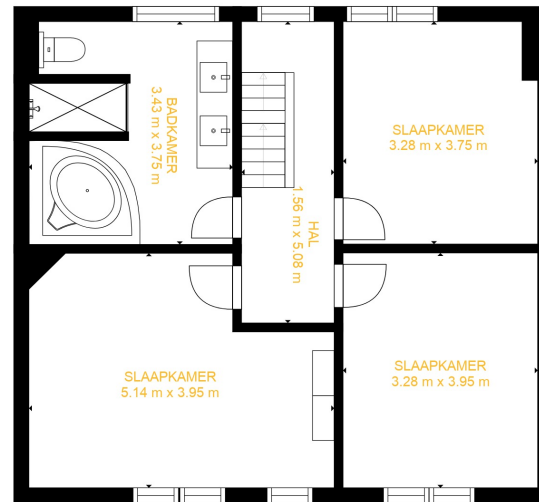
3. VERDIEPING
