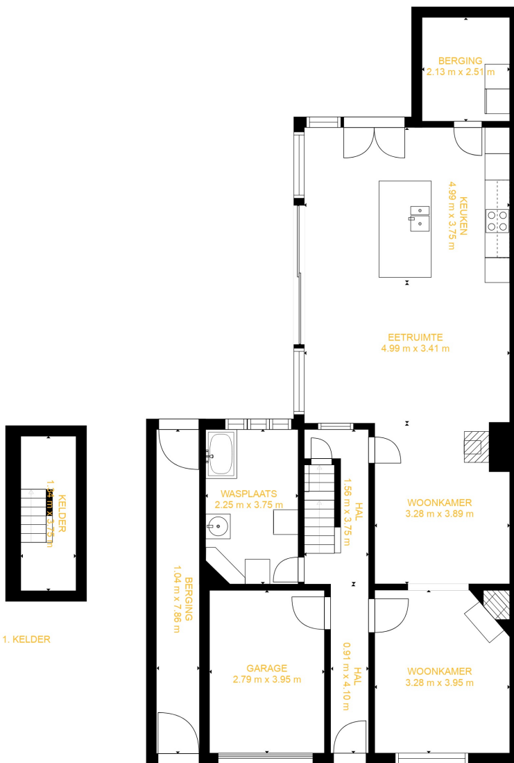
2. GELIJKVLOERS
