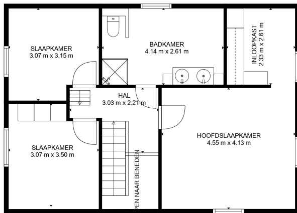
2. VERDIEPING
