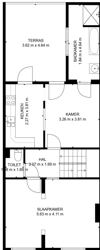
2. EERSTE VERDIEPING
