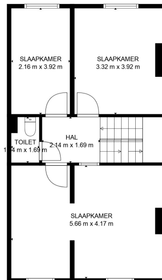
3. TWEEDE VERDIEPING
