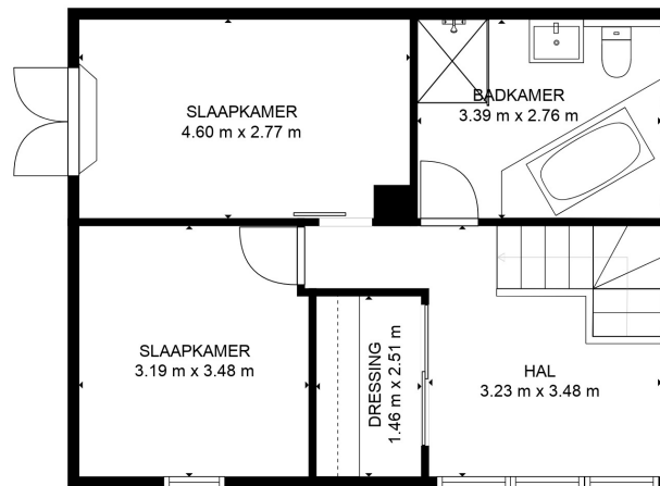
2. VERDIEPING
