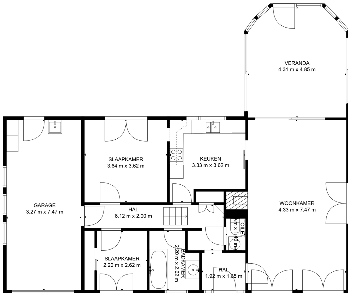
1. GELIJKVLOERS
