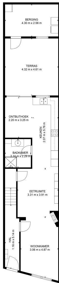
1. GELIJKVLOERS
