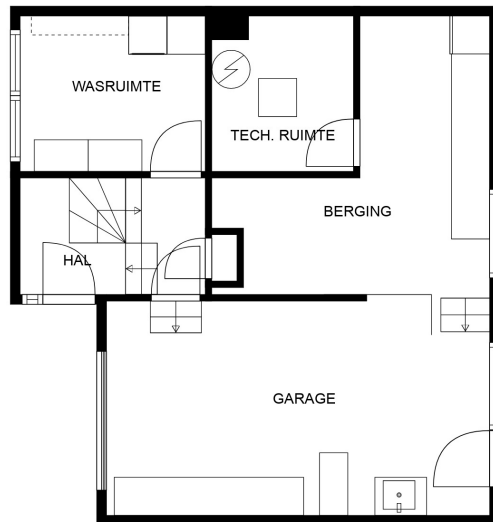
1. GELIJKVLOERS
