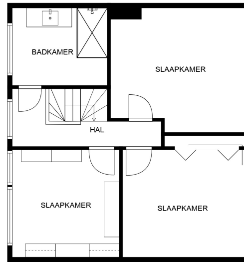
3. VERDIEPING
