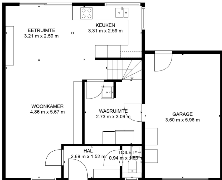
1. GELIJKVLOERS
