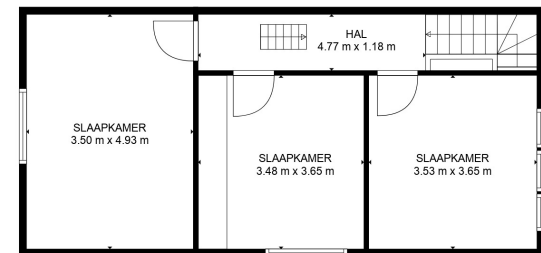
3. VERDIEPING
