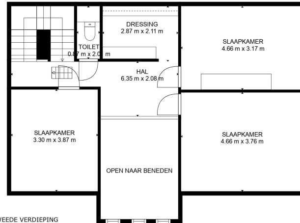
3. TWEEDE VERDIEPING
