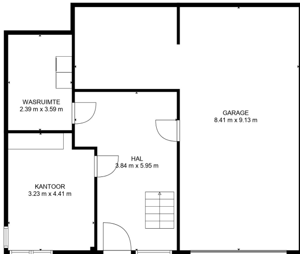
1. GELIJKVLOERS
