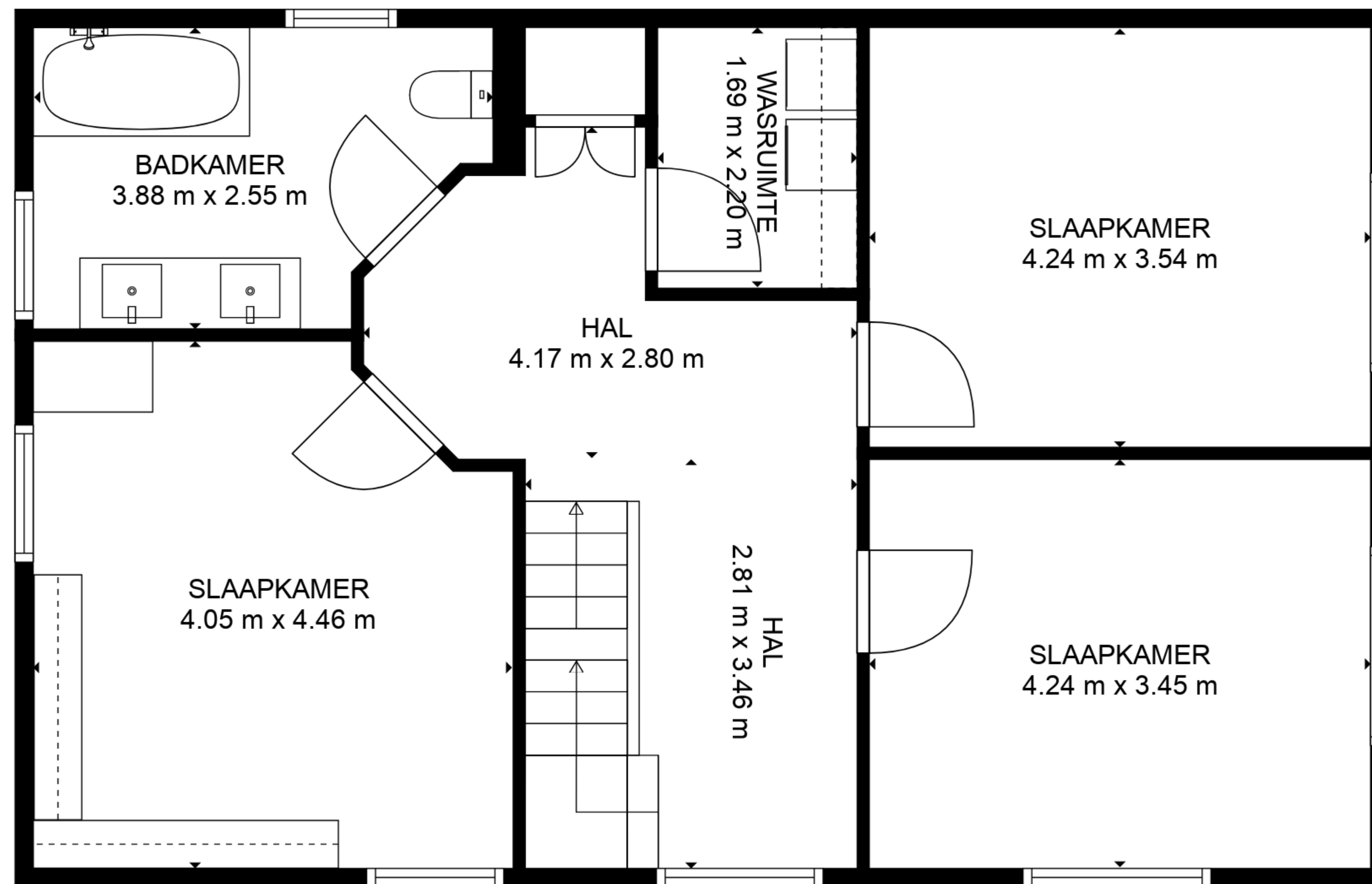
2. VERDIEPING
