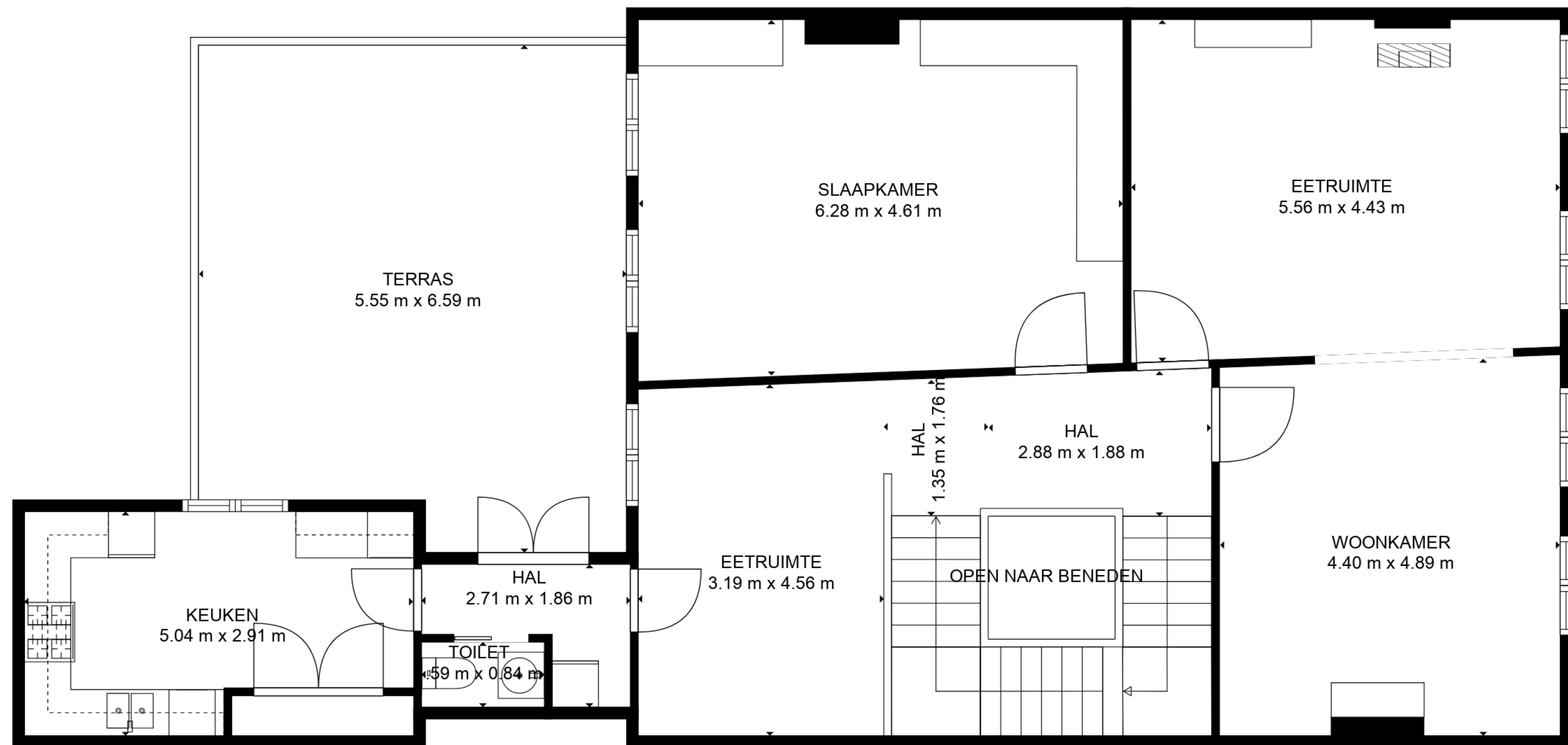
2. EERSTE VERDIEPING
