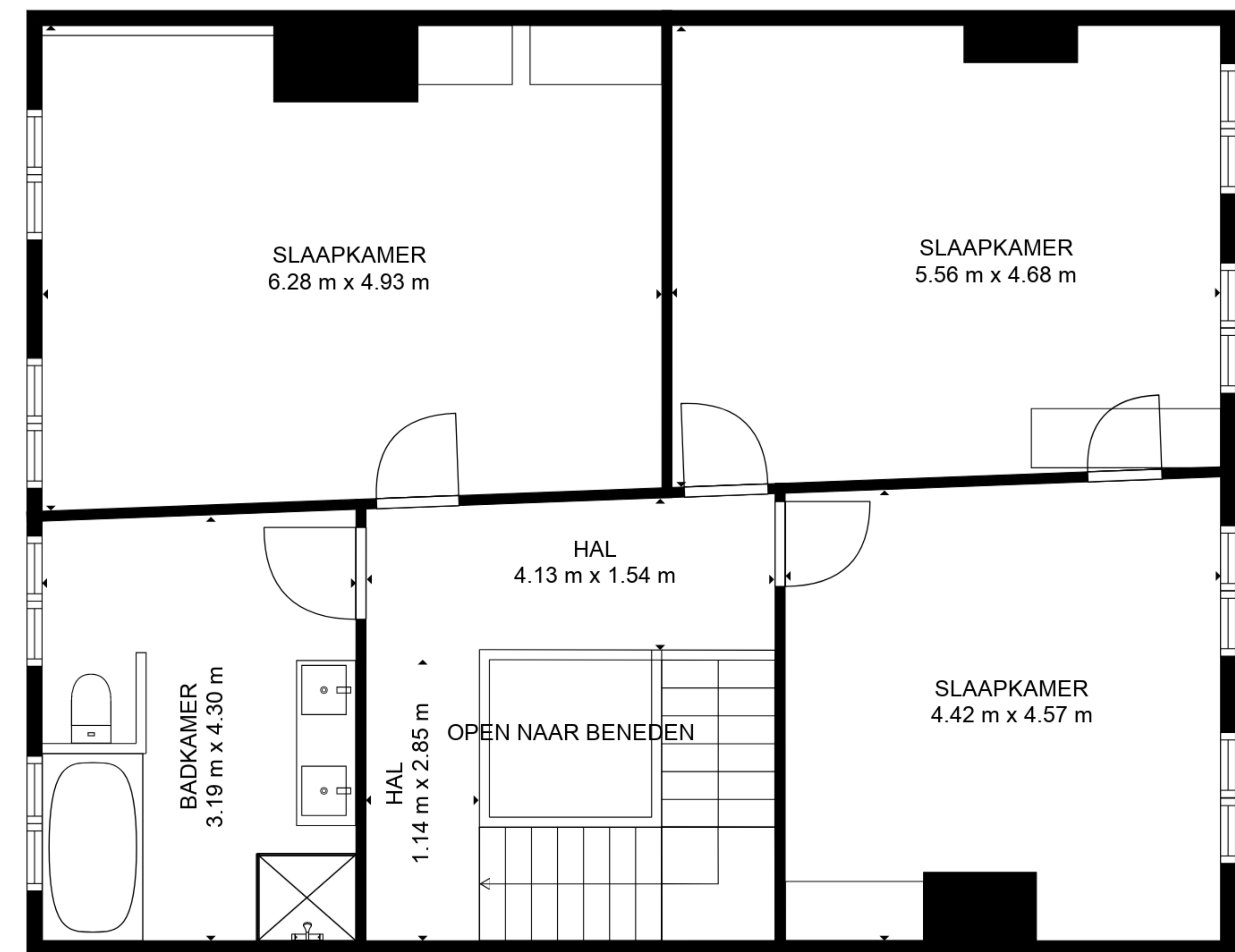
3. TWEEDE VERDIEPING
